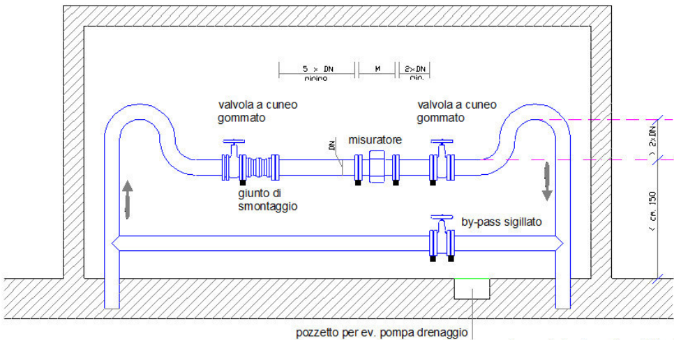
Ingombri misuratore M in funzione del diametro della tubazione
